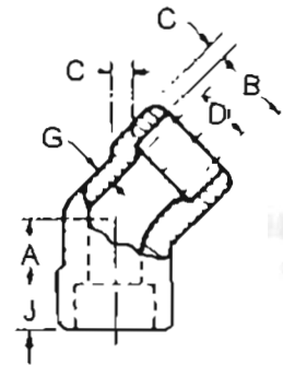
45° ELBOW
