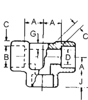
TEE
